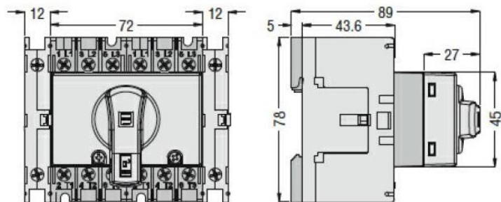
63A 4P
