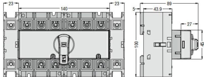
125A 4P
